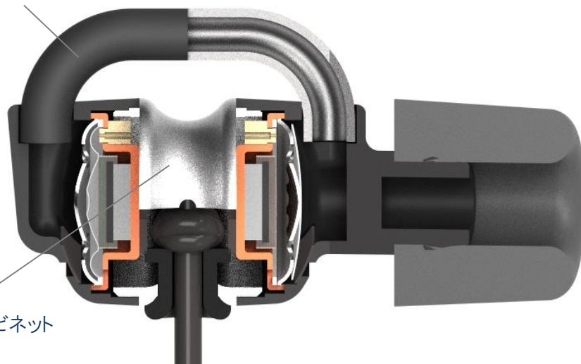
貳型制振処理位相補正チューブ
